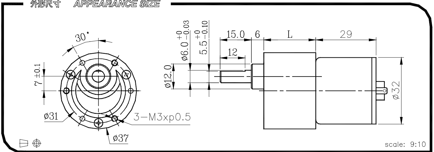
外形尺寸 APPEARANCE SIZE
